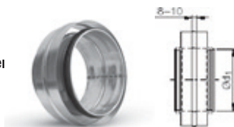
NSP50 Manicotto maschio per spessore isolamento 50 mm Male coupling
