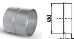
MF Manicotti di giunzione femmina Female couplings
